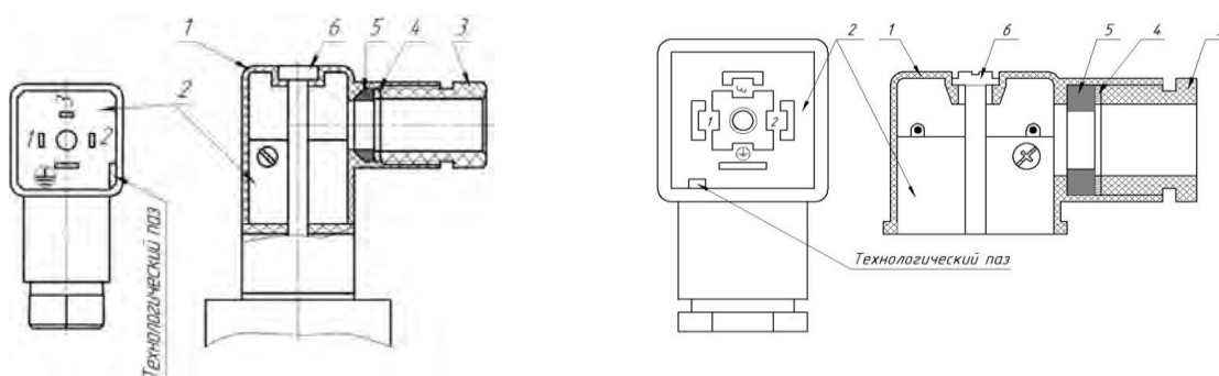
Штепсельный разъем типа DIN 175301-803 form A
