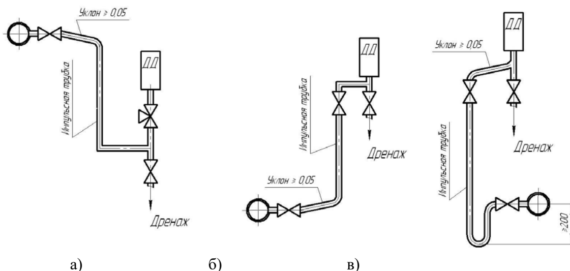
Рисунок В.3 – Установка датчика для измерения давления неагрессивной жидкости или пара при температуре выше 100^{\circ}\text{C} и P_y > 1,6 \text{ МПа} .
