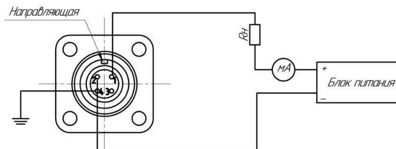
Рис. 5.4 Схема подключения датчиков, Н1
