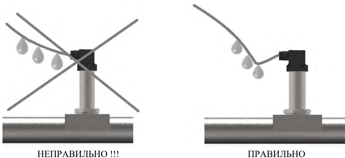
Рисунок 9.1 – Монтаж кабельного ввода
