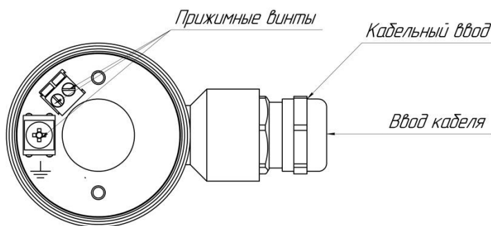
Рисунок 9.3 – Электрический разъем датчика
