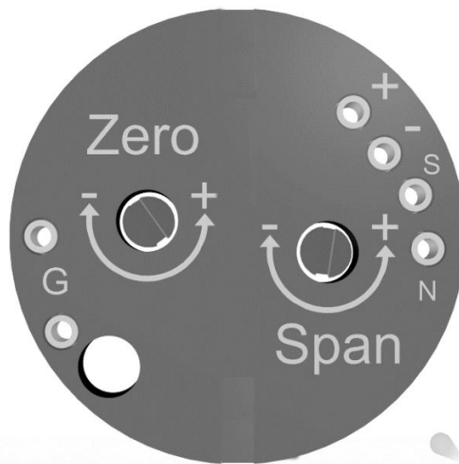
Рисунок 10.1 Интерфейс регулировки датчика
